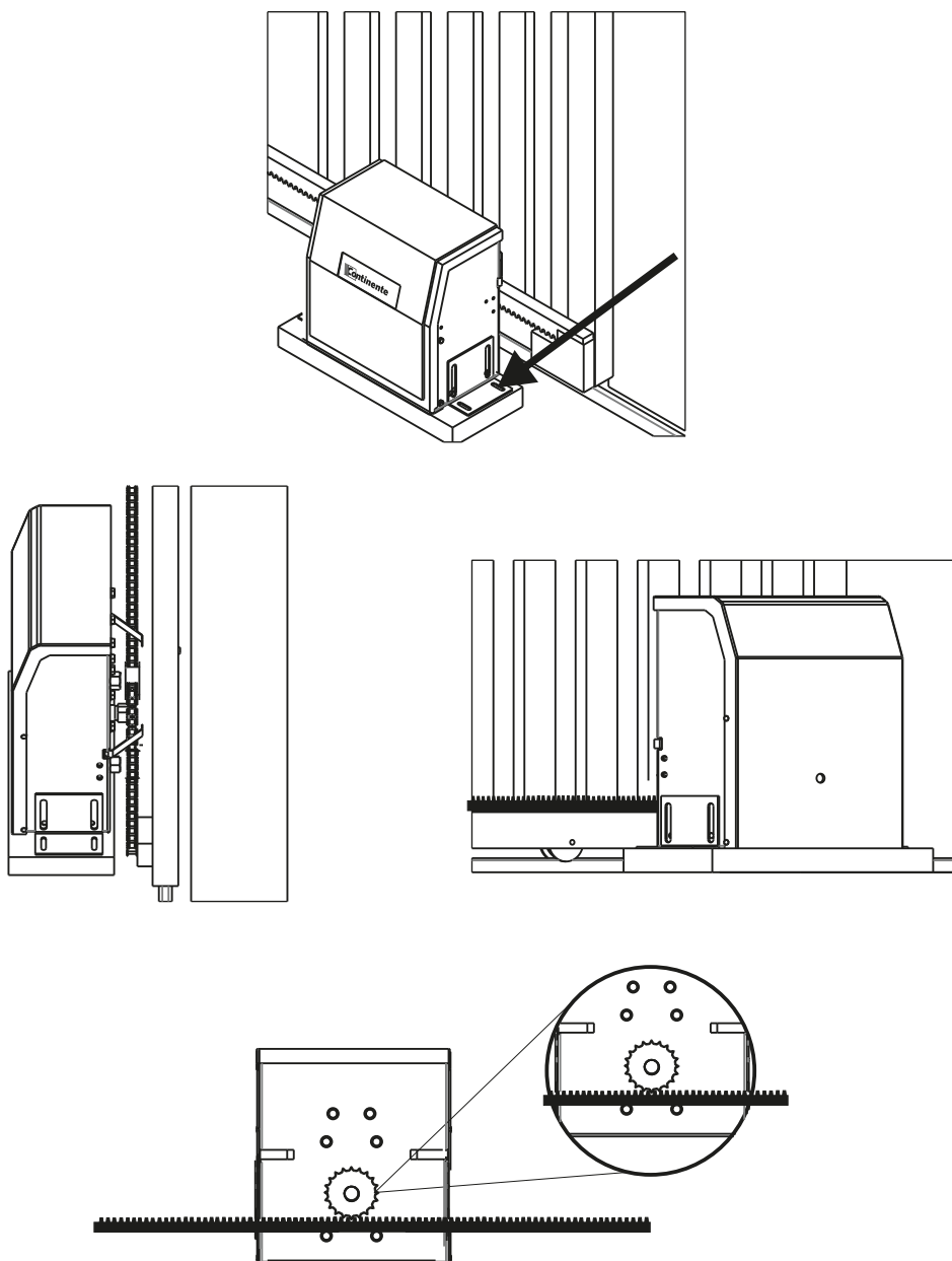
Figura 03: Fixar a cremalheira no portão, com um ponto de solda, observando que a engrenagem se encaixe na cremalheira, para que ocorra a movimentação do portão no momento que o movimentador for acionado.
